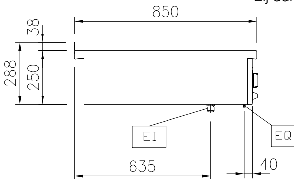
Zij aanzicht
