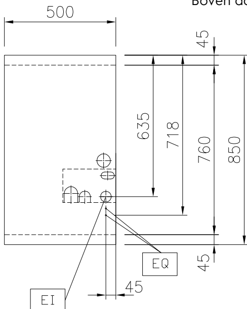
Boven aanzicht
